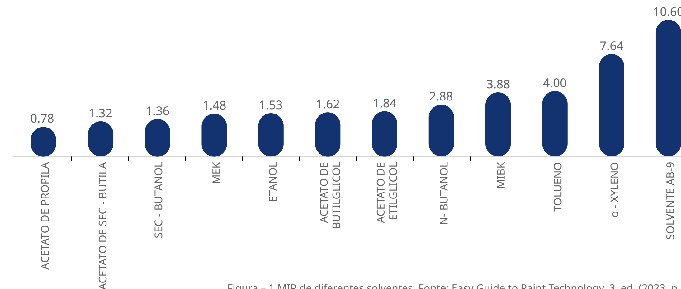
Figura – 1 MIR de diferentes solventes. Fonte: Easy Guide to Paint Technology. 3. ed. (2023, p 52).
